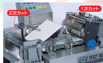
高速角切り機のスライス機構
