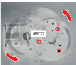
丸刃偏芯軌道 丸刃に取付穴が3箇所あり、取付位置を変更することで通常の3倍使用可能。
